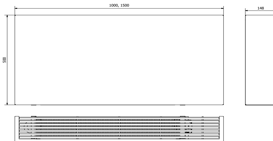
Нижнее подключение
