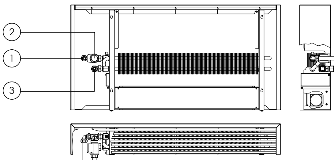
Боковое подключение
