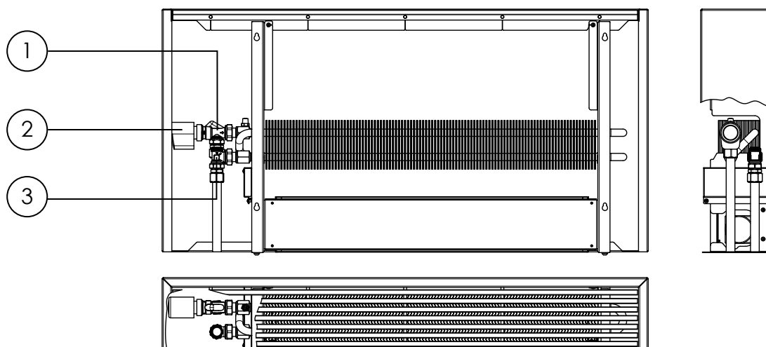
Боковое подключение
